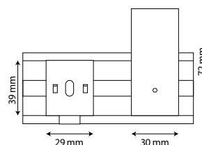
Inbouwdiepte /bovenaanzicht
